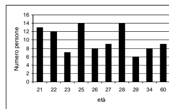
Istogramma equi-heigh
